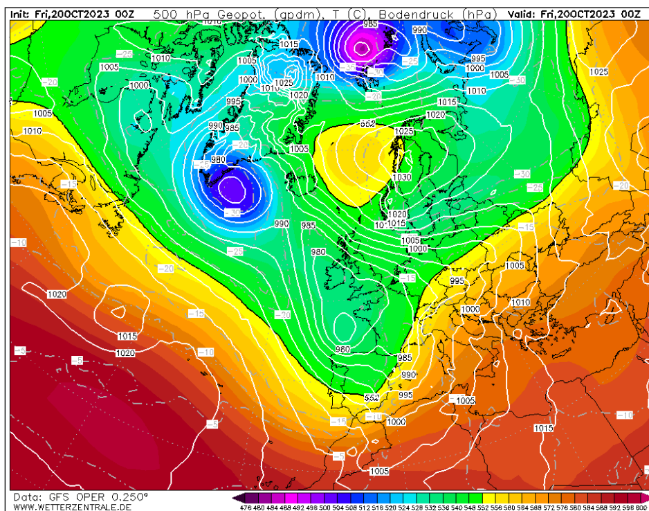
Situación sinóptica del de la noche del jueves 19 y madrugada del viernes 20-10-2023 (00Z). Geopotencial a 500 hPa y mapa de superficie.
